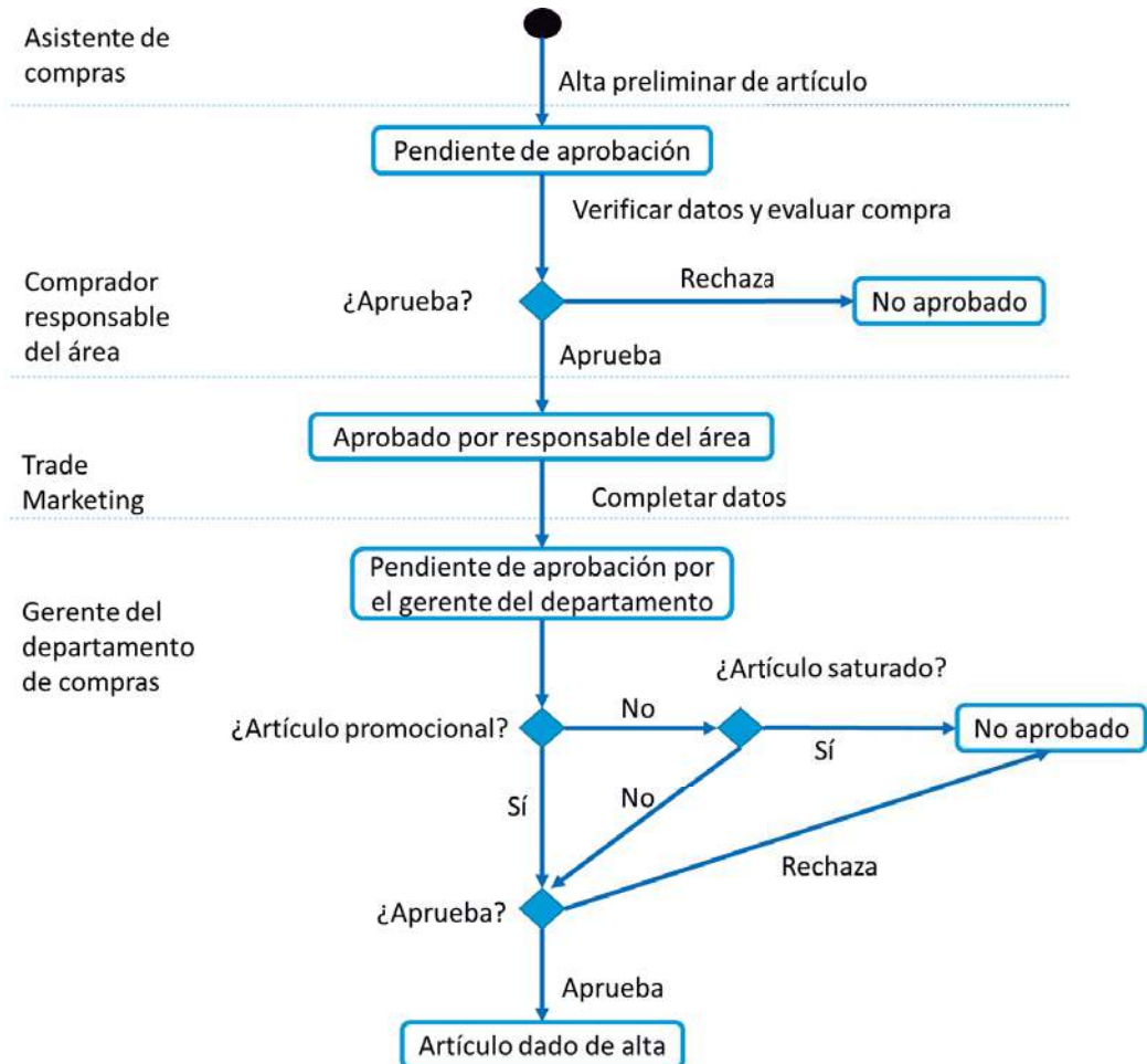
FIGURA 15 - MÁQUINA DE ESTADOS PARA SISTEMA DE GESTIÓN DE ARTÍCULOS
