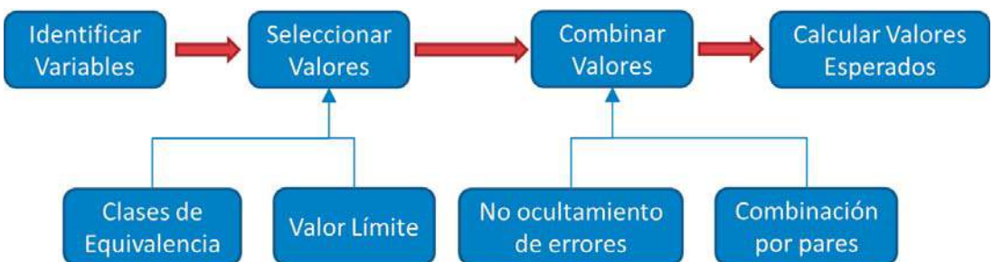
FIGURA 1 – PROCESO BÁSICO DE DISEÑO DE PRUEBAS
